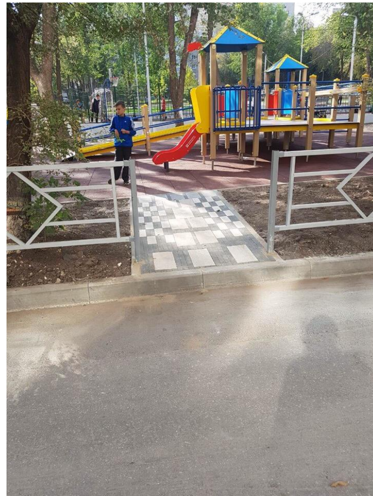
Устройство тротуара для входа на детскую площадку
